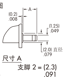
见支脚详图
