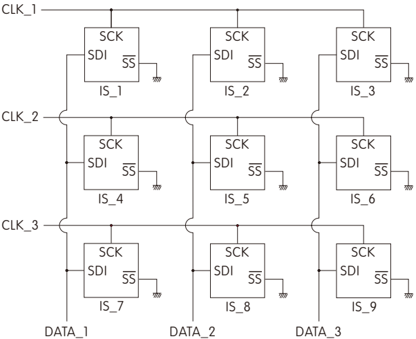
电路实例
