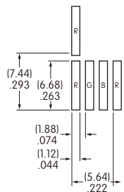
像素详图
