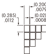
象素详图
