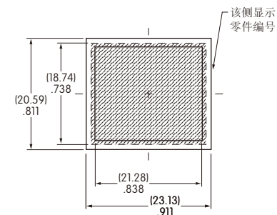
像素详图
