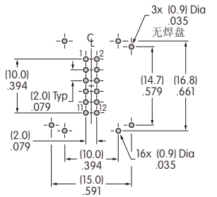
覆盖区
