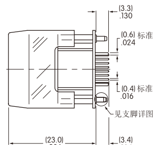
见支脚详图
