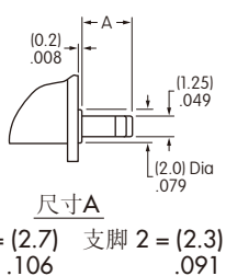
支脚详图
