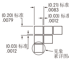
像素详图
