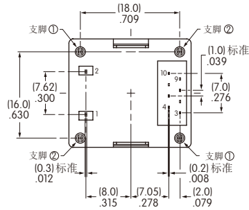
引脚足迹
