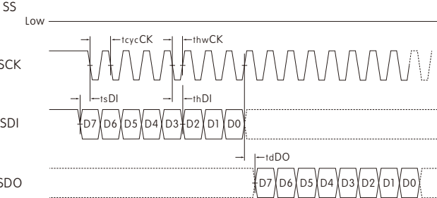
SPI 定时图（ \overline{SS} 低电平固定）
