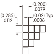
像素详图
