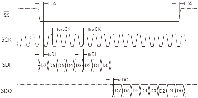
SPI 定时图（ \overline{SS} 使用）
