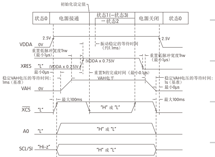
电源 ON/OFF 序列
