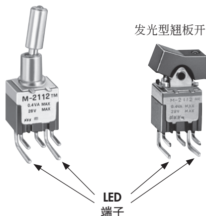
发光型拨动开关
